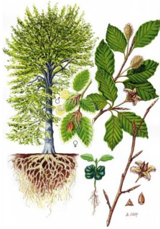
buk lesní
